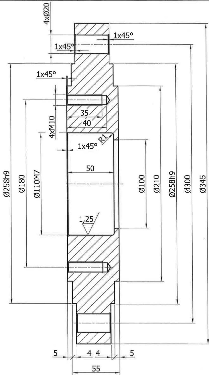
Pompa RPZ80-250W. Przedłużenie wału pompy.
